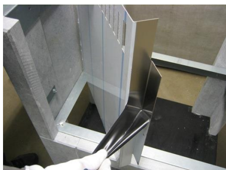
7. Poista suojamuovi takalevystä niiltä kohdin, jotka jäävät kiveä vasten
