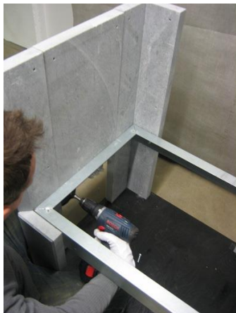
4. Sivukivet kiinnitetään keskikehykseen alapäästä
